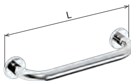
Madlo pevnostní Bath grab bar 102307012 - 355 x 55 x 75 mm 102307052 - 475 x 55 x 75 mm
