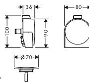
Exafill® S, vrchní sada # 58117, -000, -090, -450, -800, -810, -820, -830, -880
