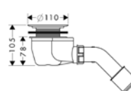
Staro® 90, zákl. těleso # 60054180
