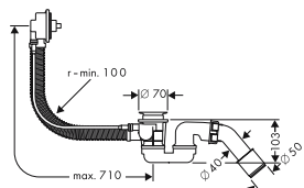
Flexaplus® ohebný, základní těleso pro zvláštní vany # 58141180
