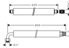
Ohebná připojovací hadice 600 mm # 58191, -000 Ohebná připojovací hadice 800 mm # 58192, -000
