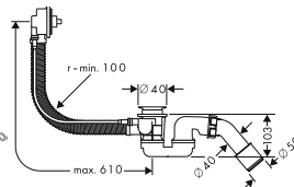
Flexaplus® ohebný, základní těleso pro normální vany # 58140180
