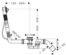
Flexaplus® pevný, základní těleso pro zvláštní vany # 58146180
