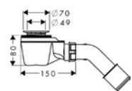
Starolift® 52, zákl. těleso # 60052180
