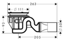
Raindrain® 90 XXL, základní těleso # 60065180
