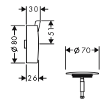
Flexaplus® S, vrchní sada # 58186, -000, -800, -810, -820, -830, -880
