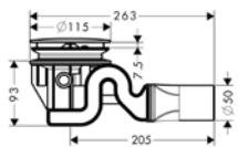
Raindrain® 90 XXL kompletní sada # 60067, -000
