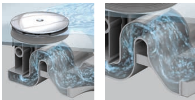
Raindrain® 90 XXL. Způsobuje to vlna v potrubí: Raindrain 90 XXL nechá v krátkém čase snadno zmizet i velké množství vody.
