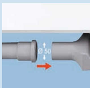
Násuvná objímka Těleso Raindrain je možné s potrubím velmi snadno spojovat díky násuvné objímce průměru 50 mm. Dosud obvyklé spojení s odtokovou trubkou v podobě šroubení je tu zbytečné.
