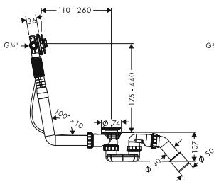
Exafill® S, základní těleso pro normální vany # 58115180
