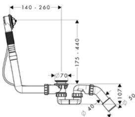
Flexaplus® pevný, základní těleso pro normální vany # 58145180
