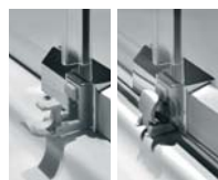
Snadná údržba: možnost vykliknutí skla
