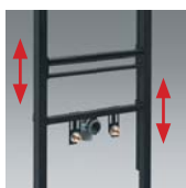
Možnost nezávislé regulace 2 příčných profilů: se šrouby pro připevnění umyvadla a s přívodními armaturami
