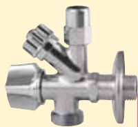
5309 Rohový ventil 1/2" x 3/4" x 3/8" pračko-roháček se zpětným ventilem
