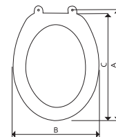
rozměry: A 440-470 mm B 380 mm C 440 mm
