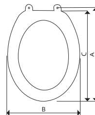
rozměry: A 420-460 mm B 380 mm C 430 mm
