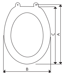
rozměry v mm: A 410-450 B 360 C 425
